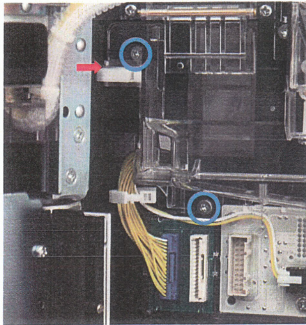
配線挟み込み対策部品を取付
