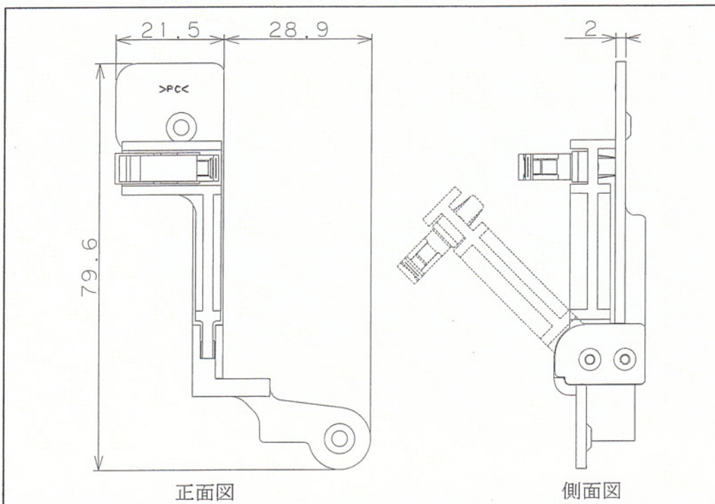
配線挟み込み対策部品の図面 (単位: mm)
