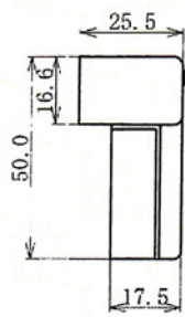
左側面図
