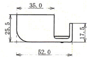
平面図
